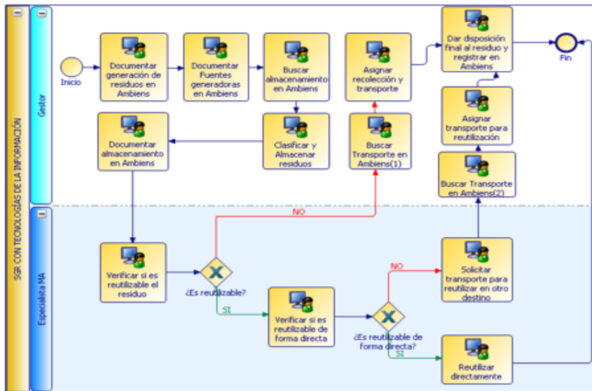
Figura 4. Proceso de aplicación del SGR hasta la disposición final con TI (imagen generada en TIBCO).
