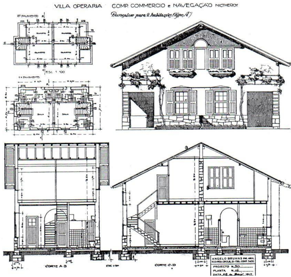
Figura 8. Chalé reunindo duas moradias. Foto: Philip Gunn, 2004; Fonte: BRUHNS, 1921, p. 50.
